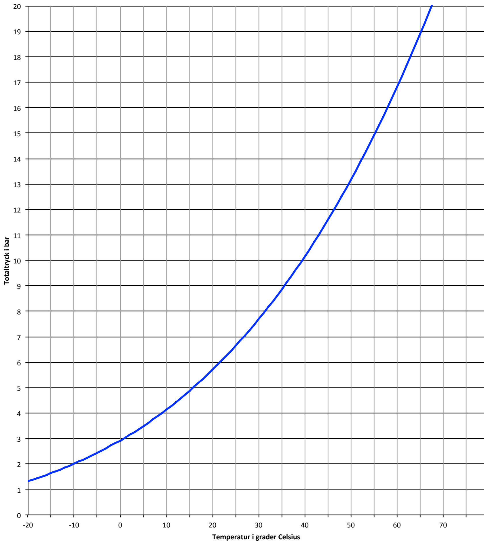
Ångtryckskurva för köldmedium R 134a
